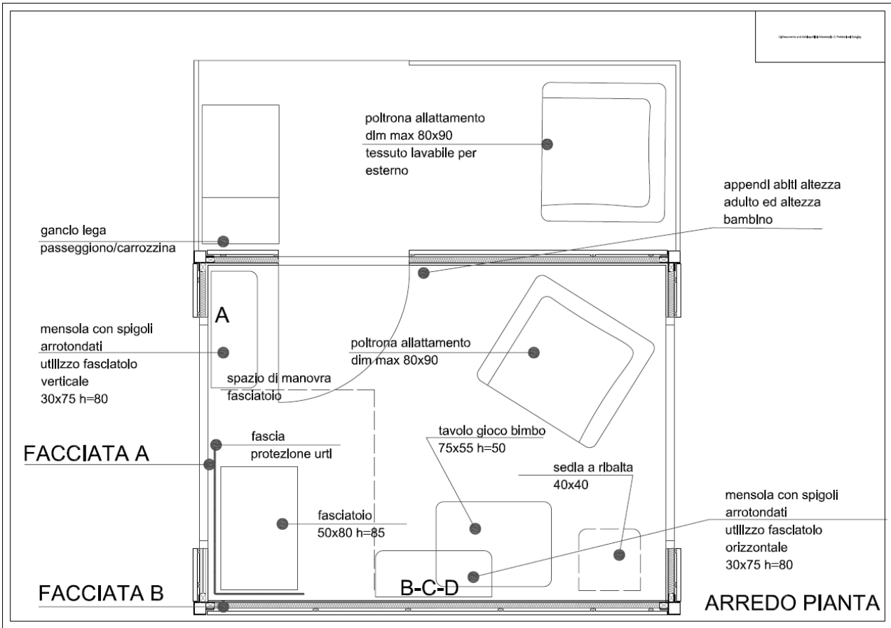
Pianta arredo
